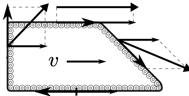
Obr. 1: Pohyb jednotlivých častí pásu: Malá šípka (vždy smeruje doprava) znázorňuje pohyb tanku vzhľadom na zem. Veľká šípka (vždy dotýčnica k pásu) znázorňuje pohyb pásu vzhľadom na tank. Ich sčítaním dostávame trojuholníkovú šípku – celkovú rýchlosť danej časti pásu vzhľadom na zem.
